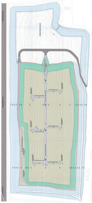
Planimetria di impianto
