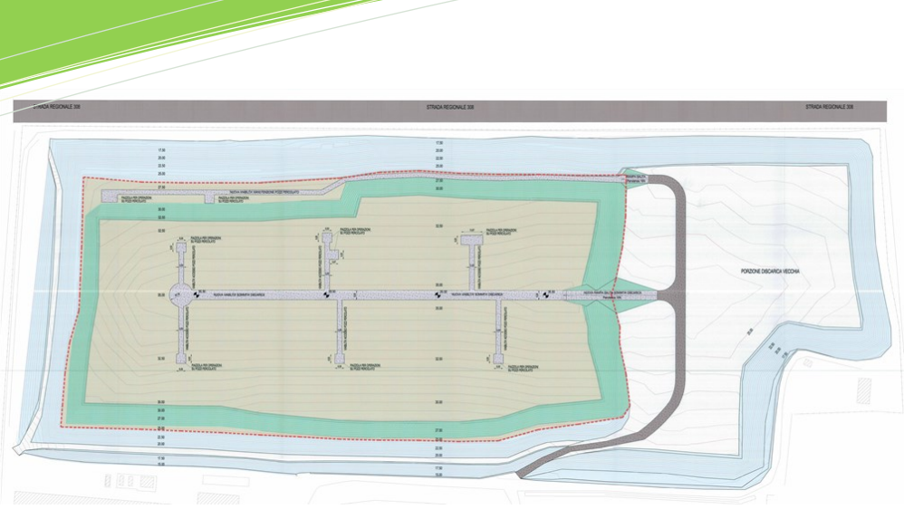
Planimetria di impianto
